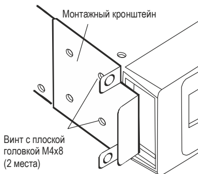
Рисунок 4 – Установка монтажных кронштейнов
