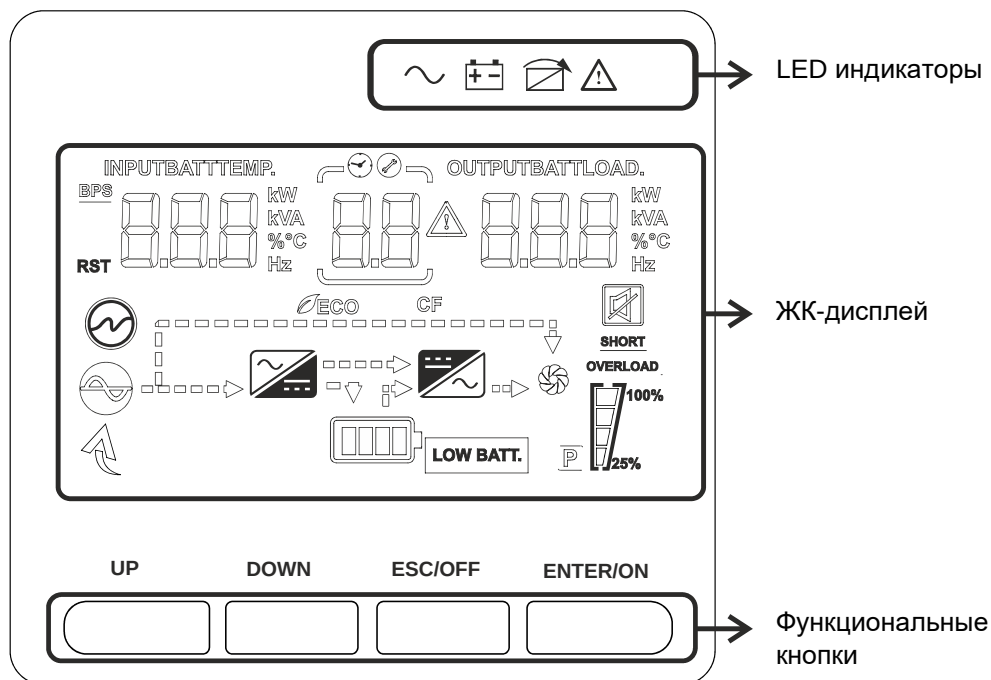
Рисунок 3 – Общий вид органов управления и индикации
