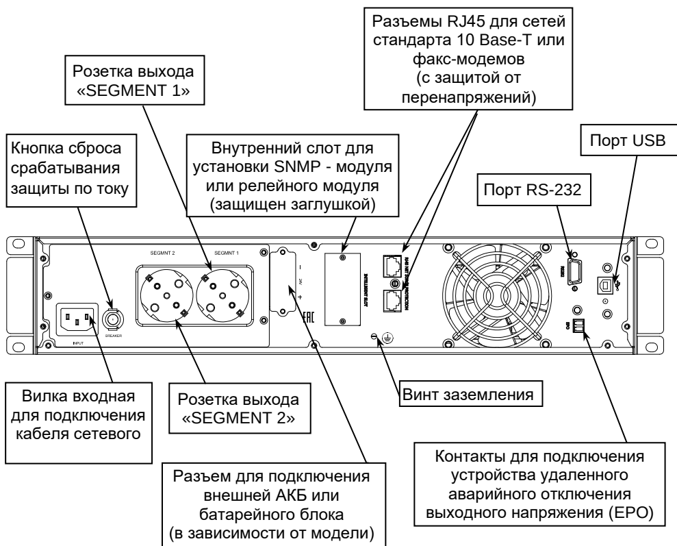
Рисунок 2 – Общий вид задней панели
