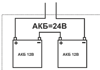
Рисунок 7 – Схема монтажа аккумуляторной батареи
